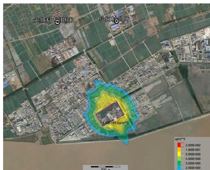
图 6.2.3-6 甲苯小时贡献浓度最大值分布
