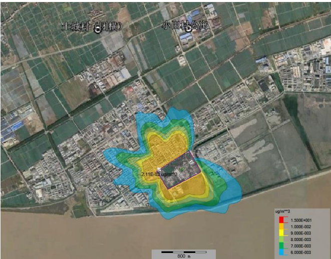
图 6.2.3-9 氯化氢日均贡献浓度最大值分布
