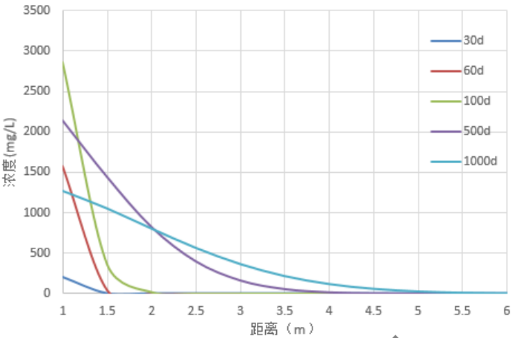
图 6.2.2-1 COD 扩散解析成果图
