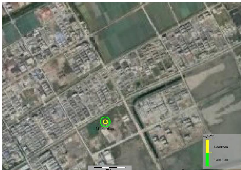
图 6.3.5-3 盐酸储罐泄漏影响预测图（最常见气象条件）
