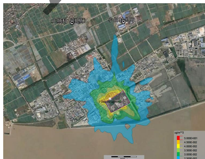
图 6.2.3-8 氯化氢小时贡献浓度最大值分布
