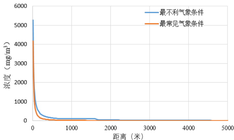
图 6.3.5-7 二氯甲烷储罐泄漏最大影响浓度与距离关系图
