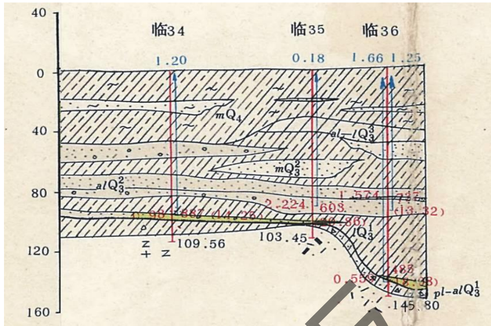
图 5.1.5-4 场址附近水文地质剖面图
