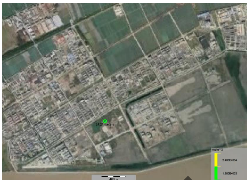
图 6.3.5-9 二氯甲烷储罐泄漏影响预测图（最常见气象条件）
