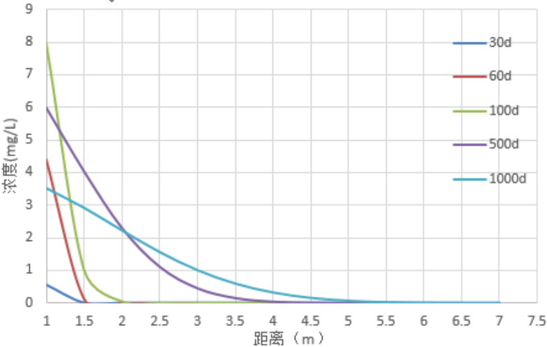
图 6.2.2-2 甲苯扩散解析成果图
