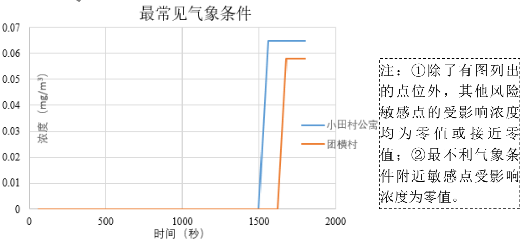
图 6.3.5-2 盐酸储罐泄漏后风险敏感点浓度随时间变化图
