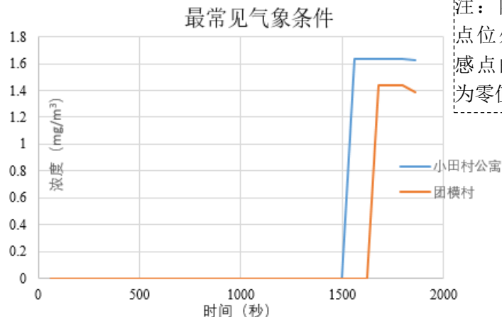
图 6.3.5-12 甲苯储罐燃烧后敏感点一氧化碳浓度与时间关系图
