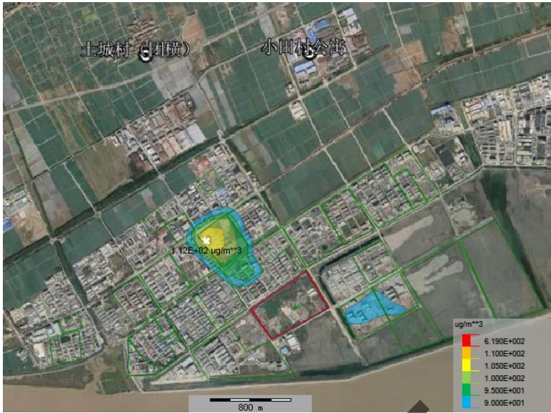
图 6.2.3-14 叠加后二氯甲烷日均预测分布图
