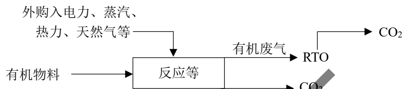
图 6.4.3.5-1 本项目二氧化碳产排节点图
